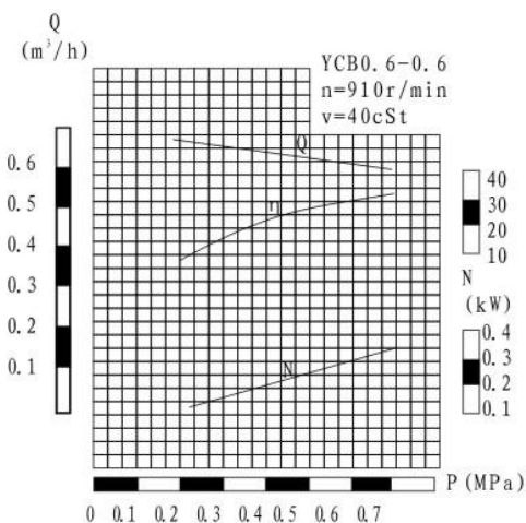
YCB 0.6-0.6型性能曲线图
