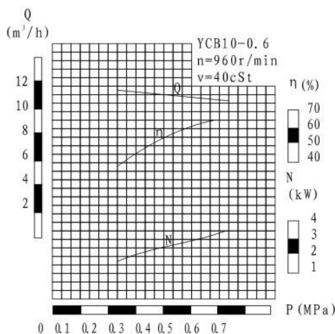
YCB 10-0.6型性能曲线图
