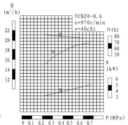
YCB 20-0.6型性能曲线图
