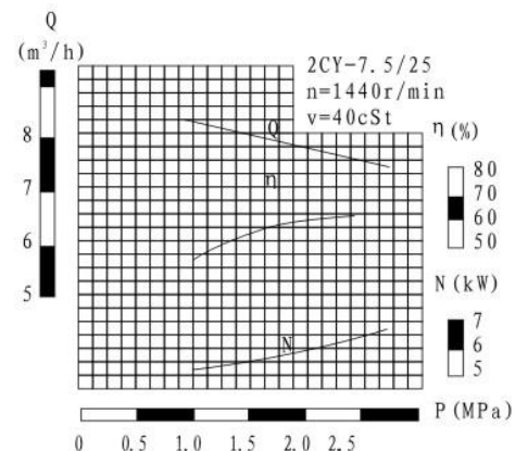
2CY-7.5/25型性能曲线图
