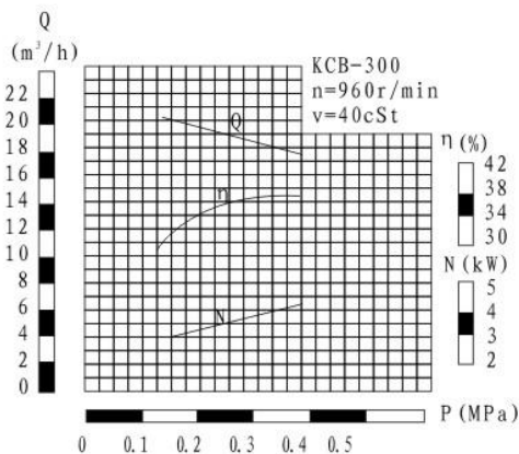
KCB-300型性能曲线图
