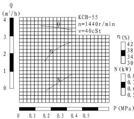
KCB-55型性能曲线图
